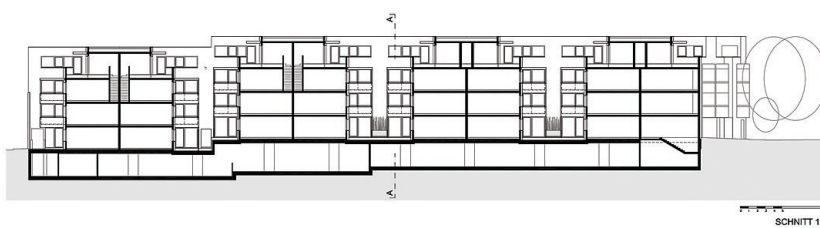
Schnitte
