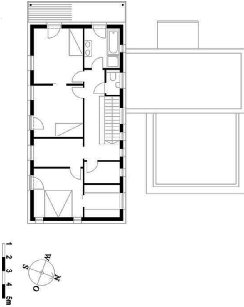
Grundriss OG
