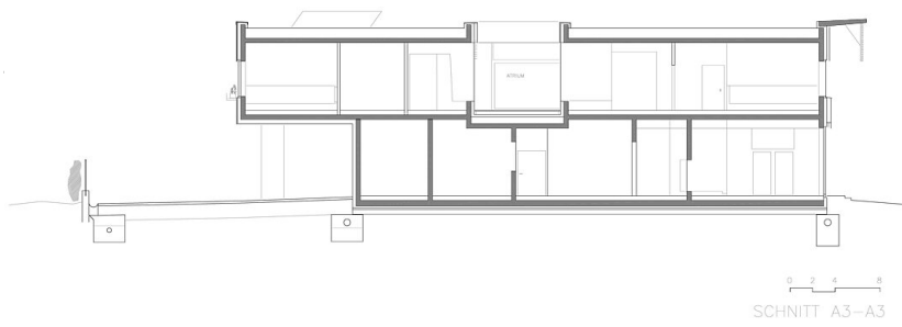
Schnitt
