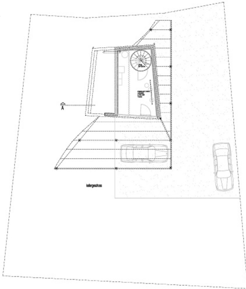
Grundriss KG
