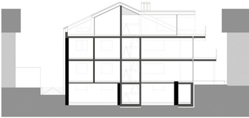
Schnitt
