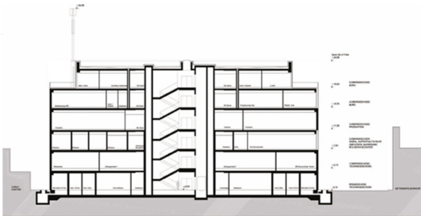
LÄNGSSCHNITT
