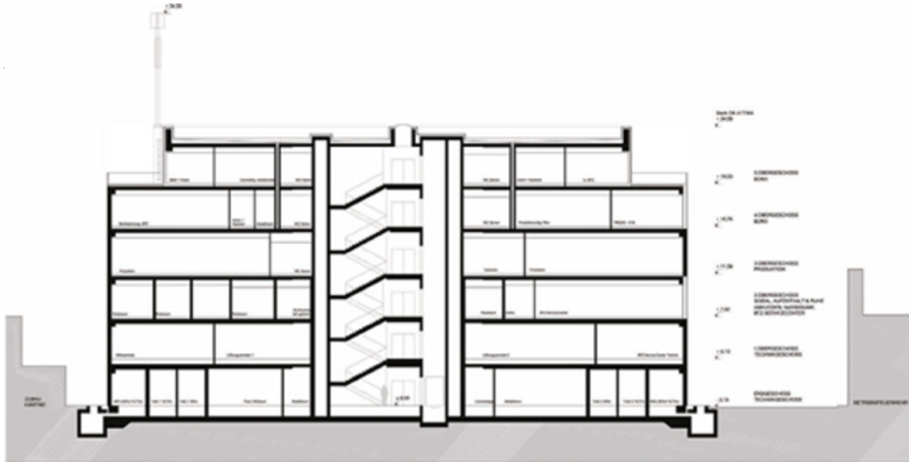
LÄNGSSCHNITT
