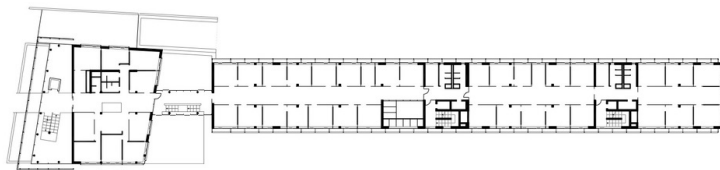
3.OBERGESCHOSS / LAENGSSCHNITT
