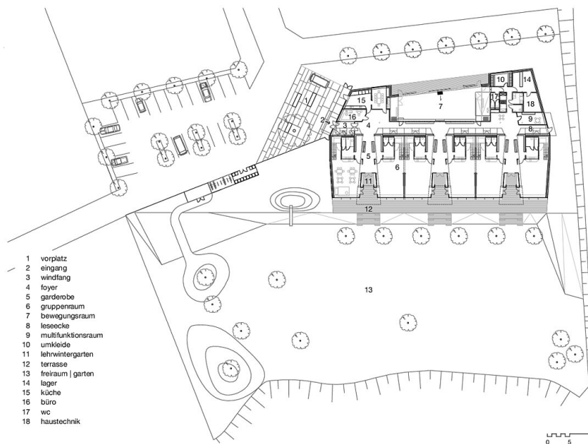
Grundriss Ebene 0
