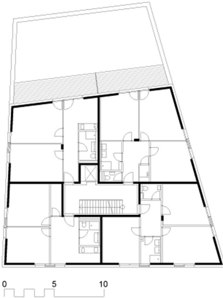
Grundriss OG
