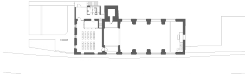
OBERGESCHOSS
