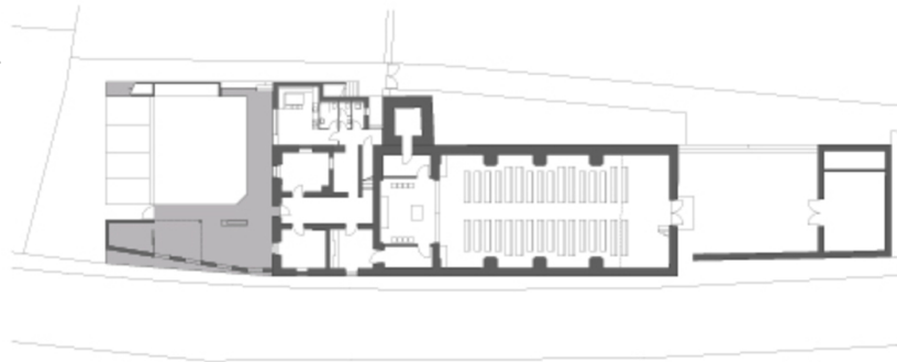
ERDGESCHOSS
