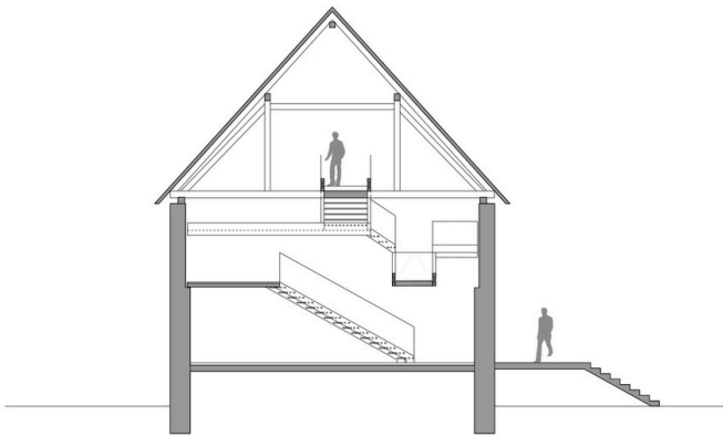
SCHNITT
