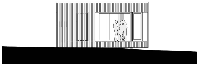
Westansicht
