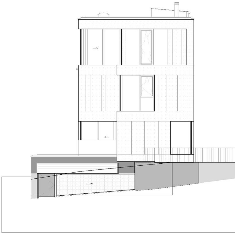
Ansicht Nord
