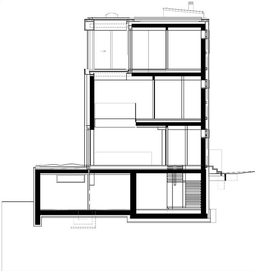
Schnitt B1-B1
