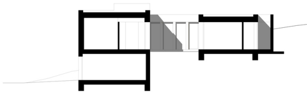
LÄNGSSCHNITT
