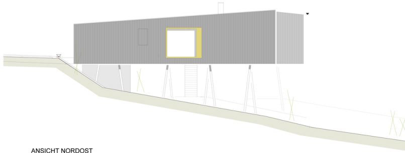
ANSICHT NORDOST
