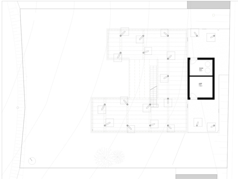
Grundriss UG
