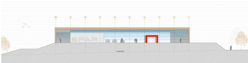
Ansicht Nord
