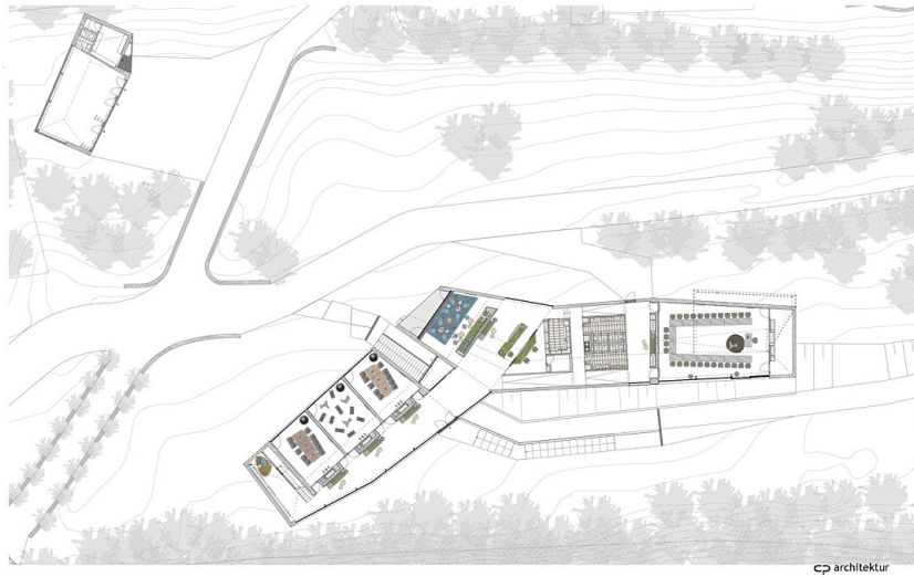
Grundriss EG III+IV
