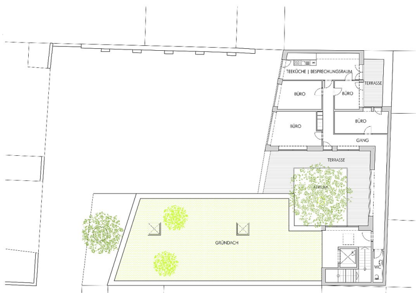
Grundriss Obergeschoss
