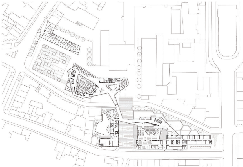
Grundriss Boulevardebene
