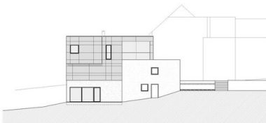
ANSICHT NORD
