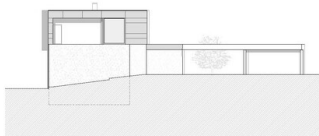
ANSICHT WEST
