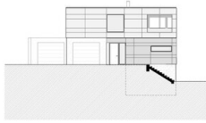
ANSICHT SÜD
