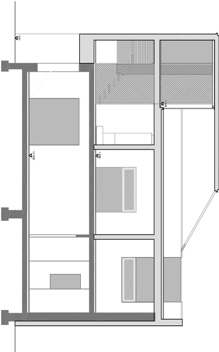
Schnitt
