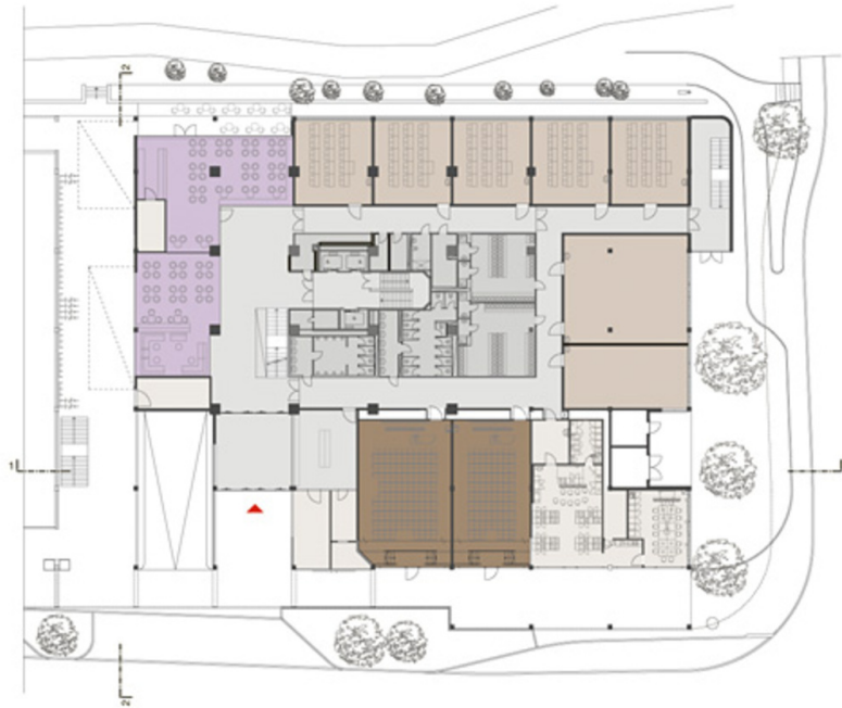
Grundriss EG
