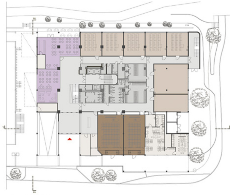
Grundriss EG
