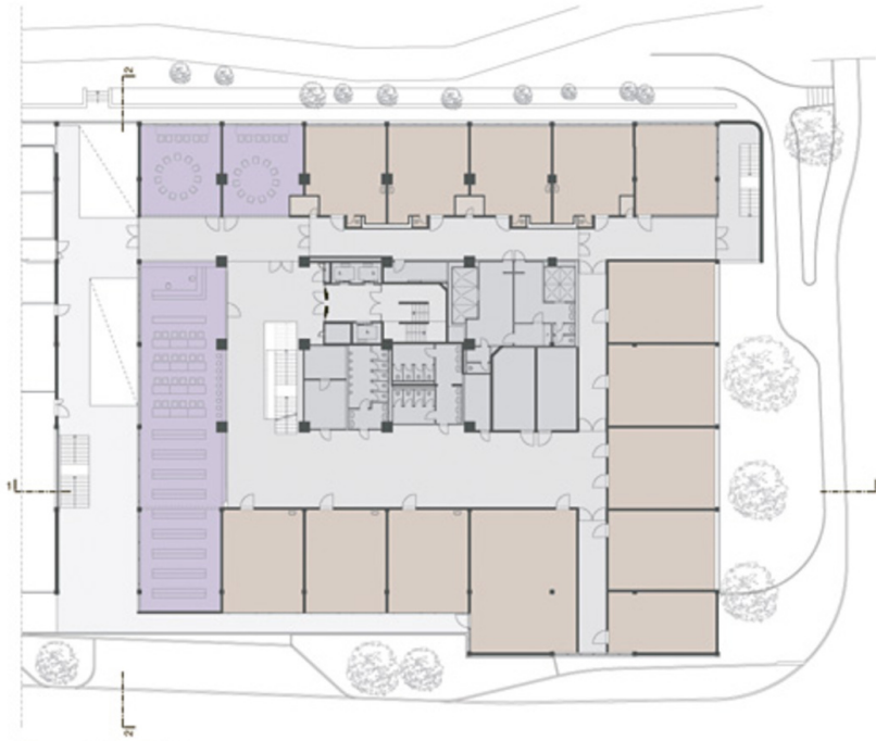
Grundriss OG1
