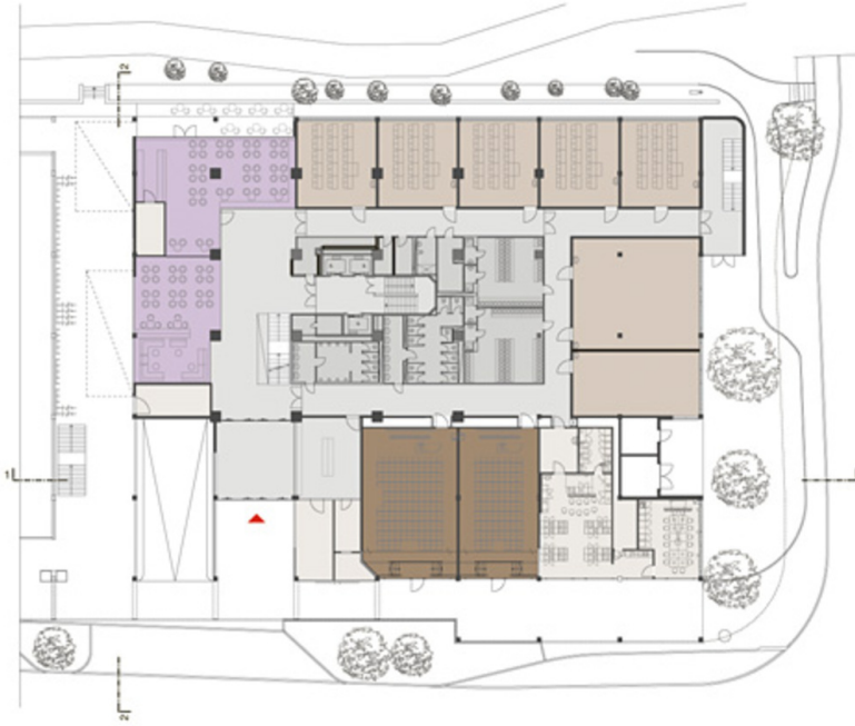
Grundriss EG
