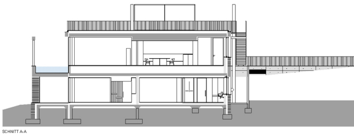
SCHNITT A-A
