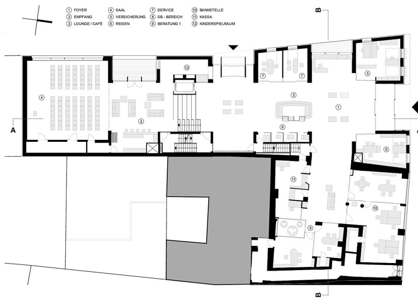
Grundriss Erdgeschoss
