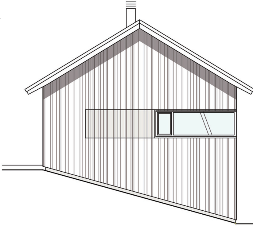
Ansicht Nordost
