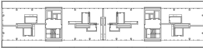
Wohnhochhaus Hirzenbach
