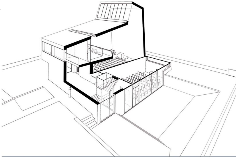
Schnitt B
