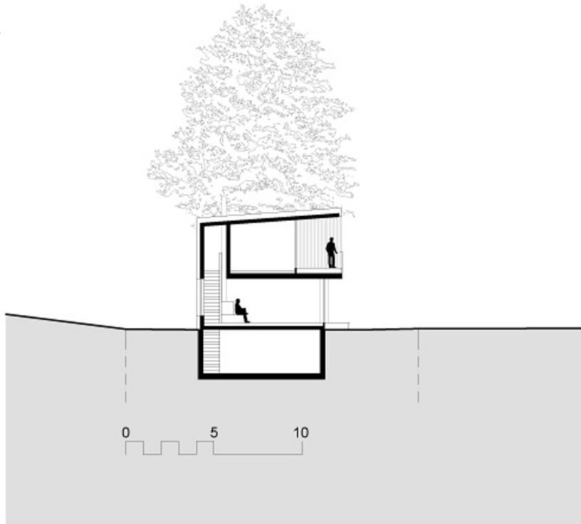
Querschnitt
