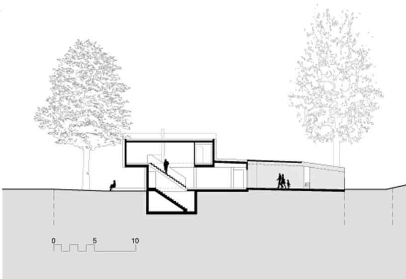
Längsschnitt
