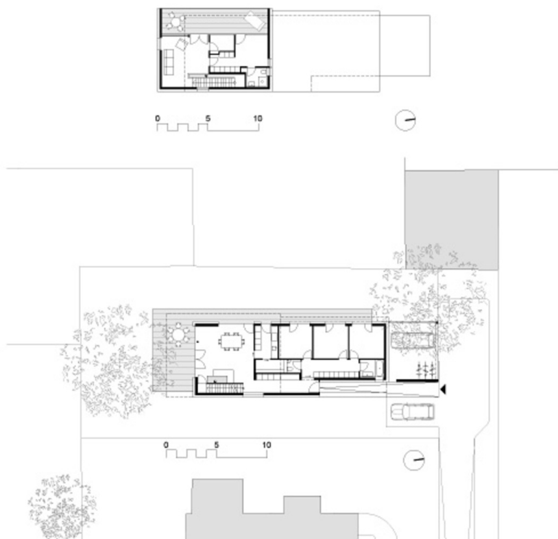
Grundriss
