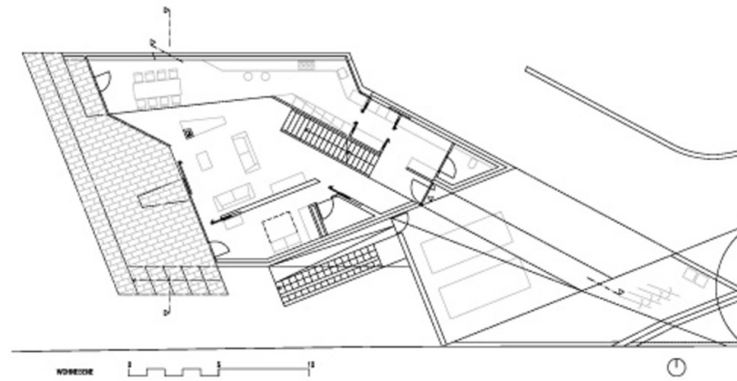
Grundriss
