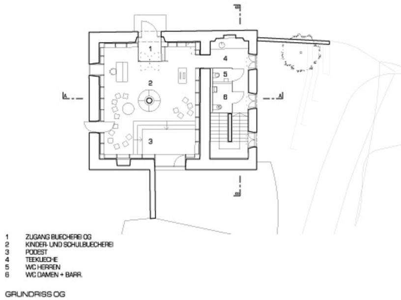
GRUNDRISS OG
