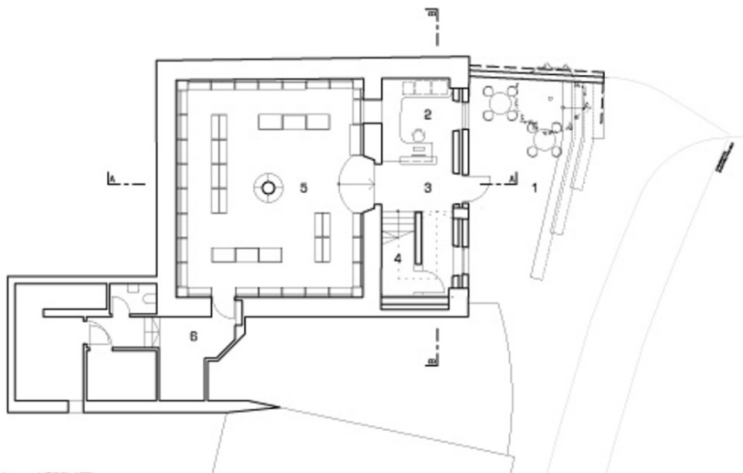
GRUNDRISS OG
