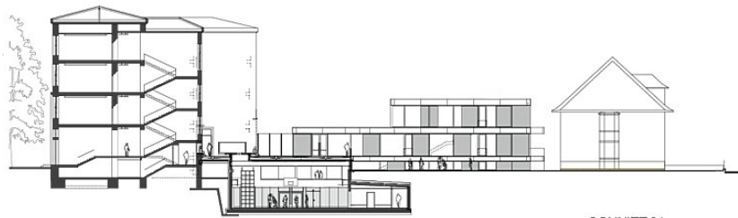
SCHNITT 01
