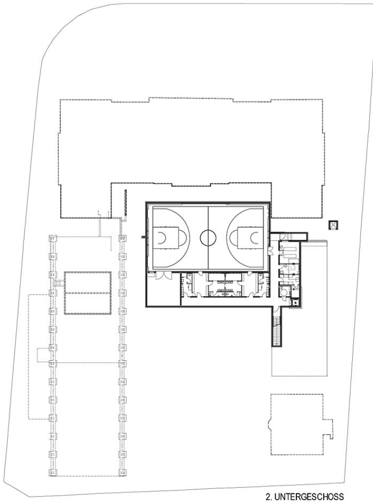
2. UNTERGESCHOSS
