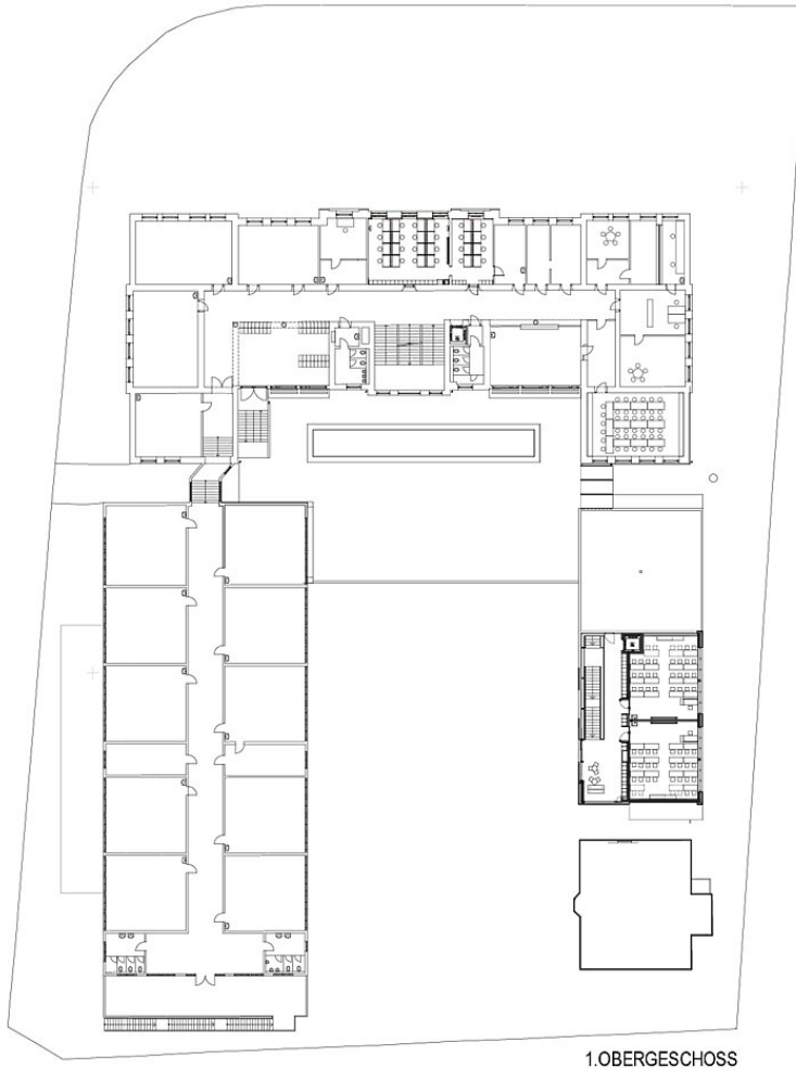
1.OBERGESCHOSS
