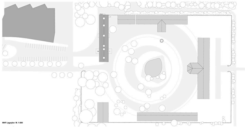
MHF Lageplan M. 1:500
