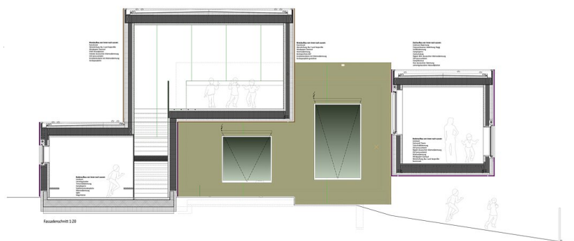
Fassadenschnitt
