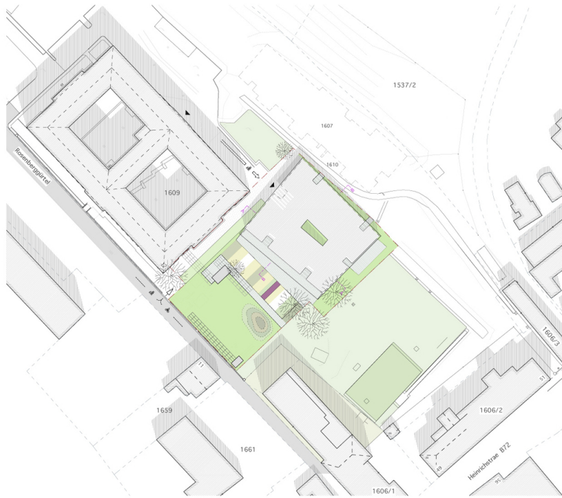
① LAGEPLAN M 1:500
