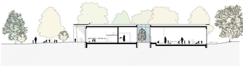
SCHNITT QUER B-B M 1:200
