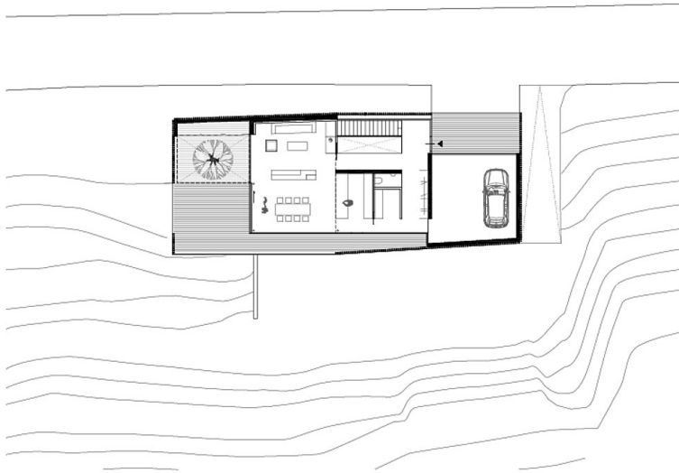
Erdgeschoß
