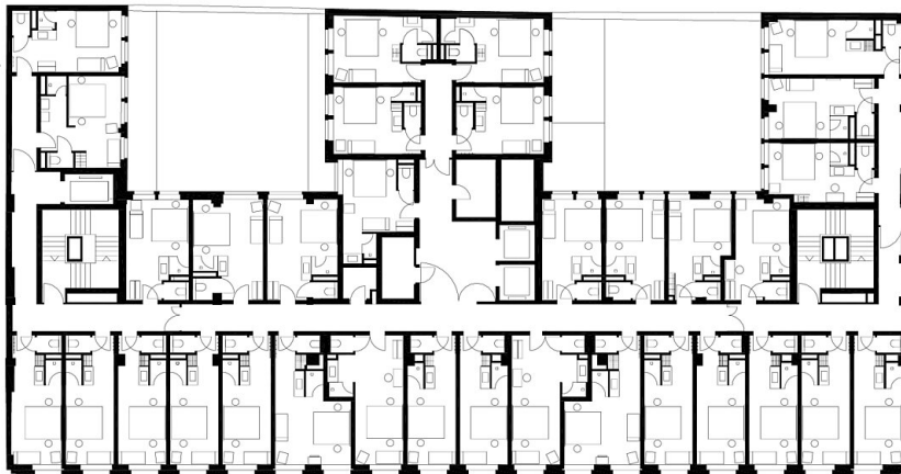
Grundriss 3. Obergeschoss
