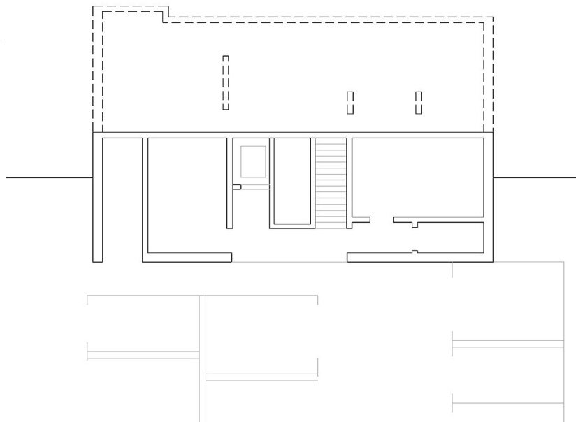
Grundriss Sockelgeschoss
