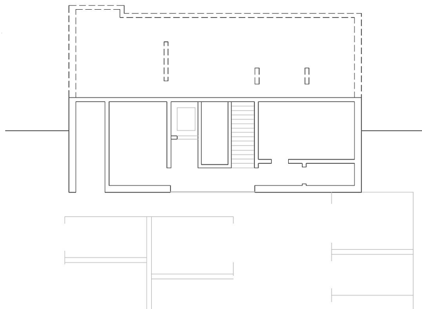
Grundriss Sockelgeschoss
