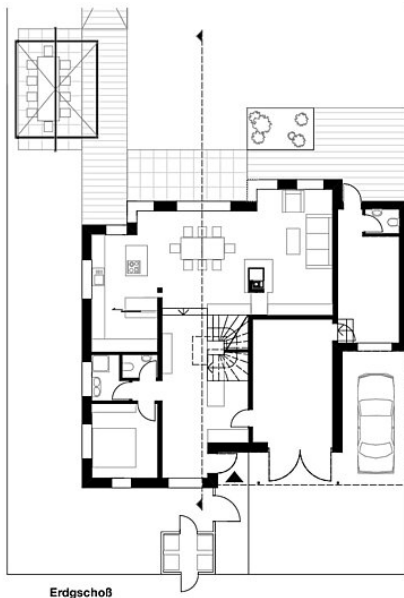
Erdgeschoß
