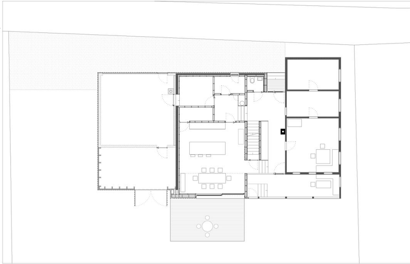
Erdgeschoß
