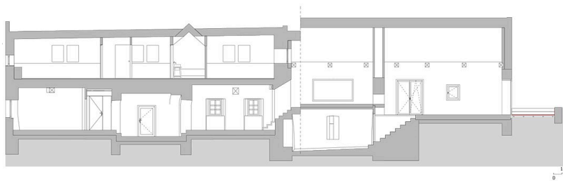
Schnitt Haus
