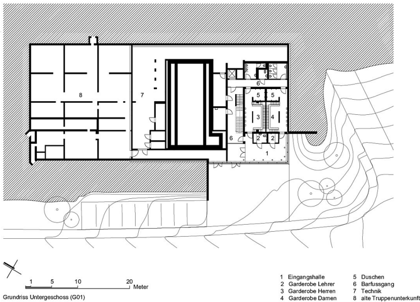
Grundriss UG
