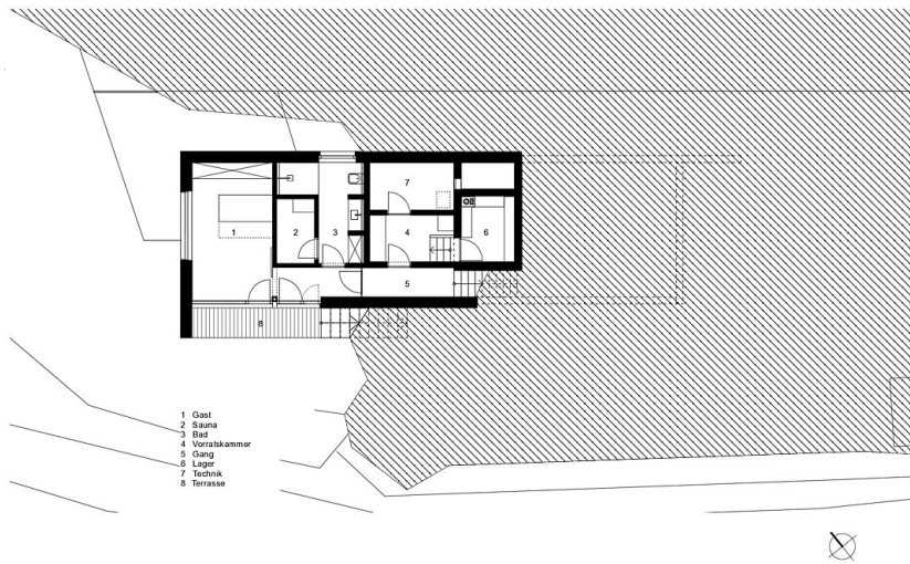
HAUS NHG GRUNDRISS UNTERES GESCHOSS M 1:100
