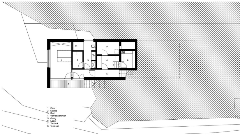
HAUS NHG GRUNDRISS UNTERES GESCHOSS M 1:100
