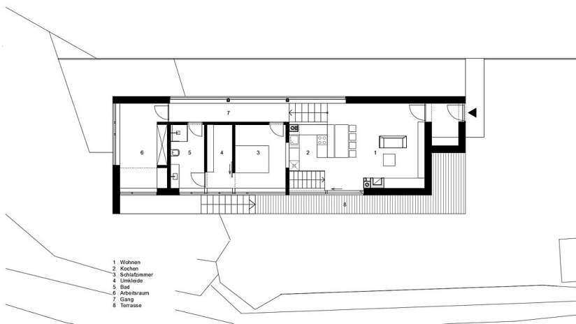
HAUS NHG GRUNDRISS OBERES GESCHOSS M 1:100
