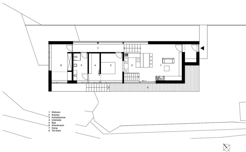
HAUS NHG GRUNDRISS OBERES GESCHOSS M 1:100
