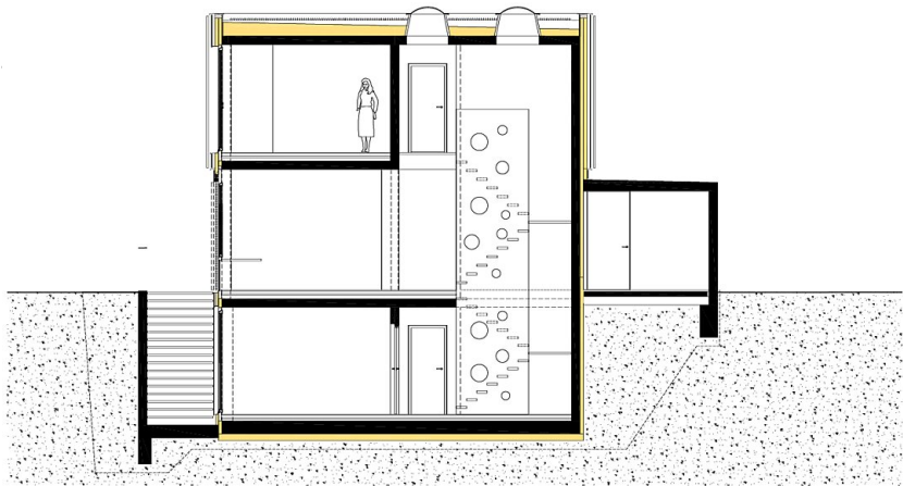
Schnitt AA
