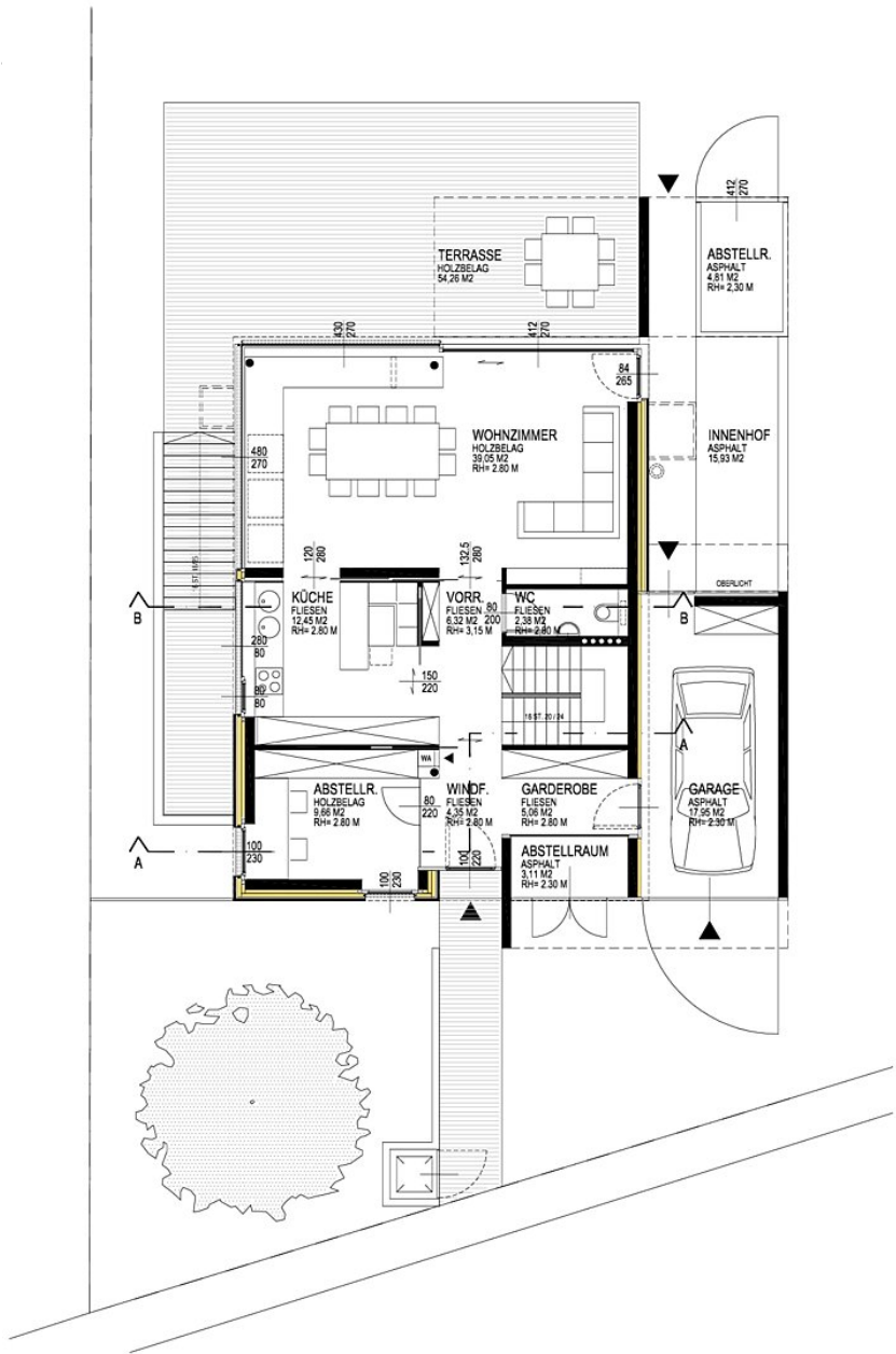
Grundriss EG
