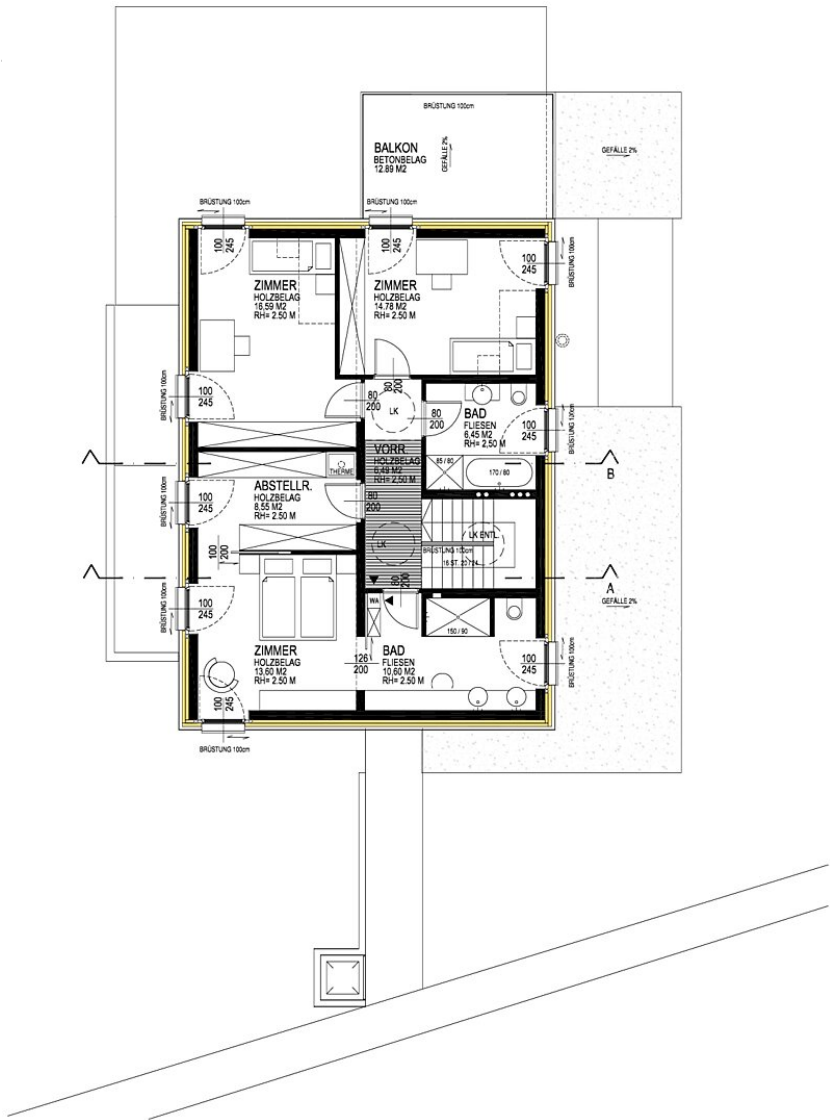
Grundriss OG
