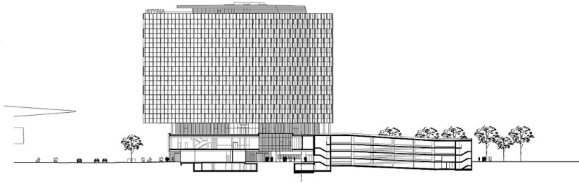
Schnitt O-W
