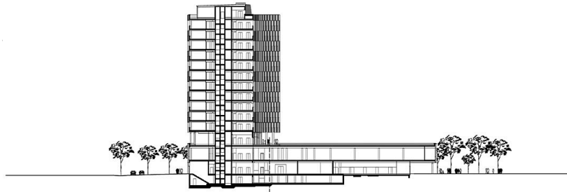
Schnitt N-S
