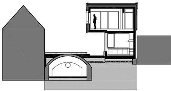
QUERSCHNITT
