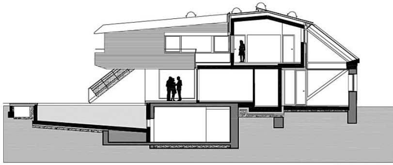
LÄNGSSCHNITT
