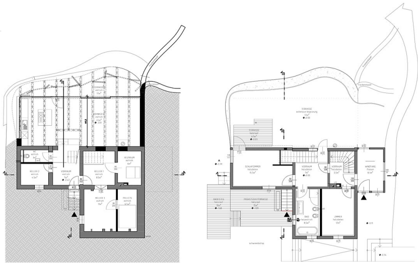
Grundriss Unteres Erdgeschoss
