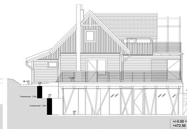
Ansicht West
