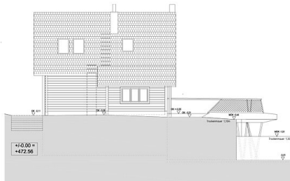
Ansicht Nord
