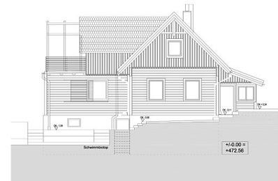
Ansicht Ost
