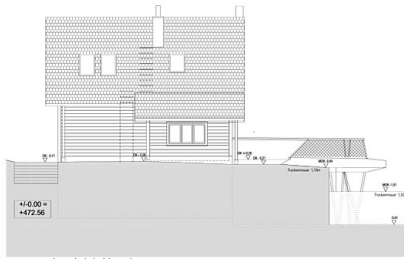
Ansicht Nord
