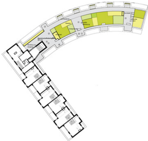
6. OG M 1:500
