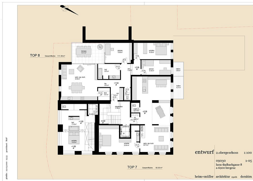
Grundriss 2. Obergeschoss
