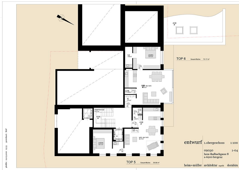
Grundriss 1. Obergeschoss
