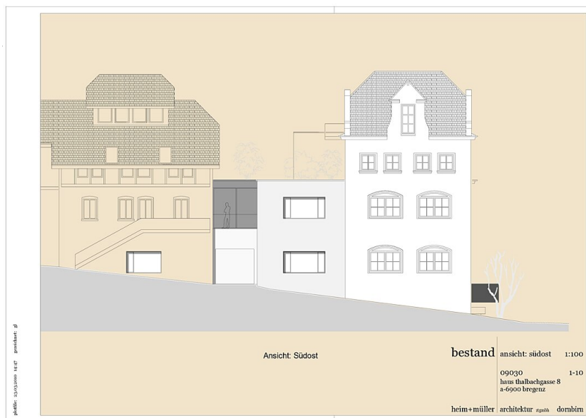
Ansicht Südost
