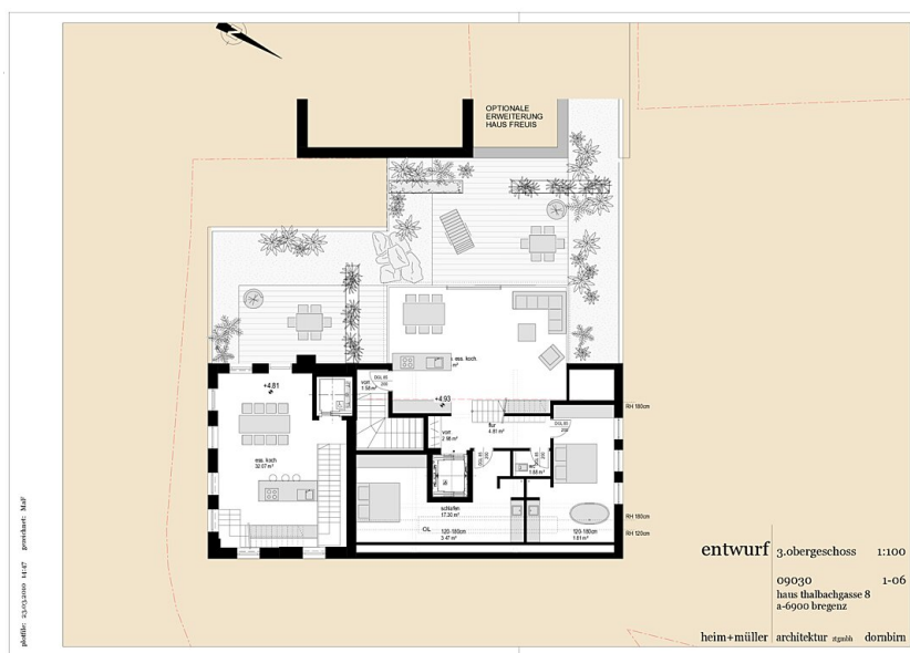
Grundriss 3. Obergeschoss
