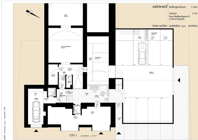
Grundriss Kellergeschoss
