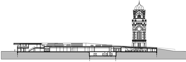
QUERSCHNITTE
