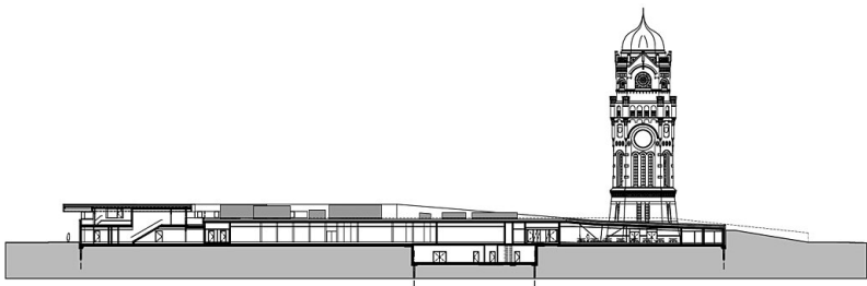
QUERSCHNITTE
